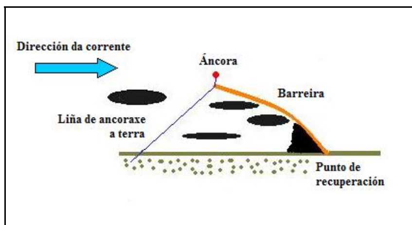
Colocación de barreiras para desviar o hidrocarburos ata unha zona de recolección
